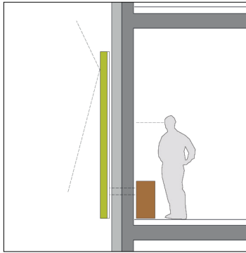
Abb. 10 Licht- und luftundurchlässige Fassadenbegrünung vor opaker Wand (THN-AR)
