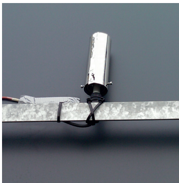
Abb. A11 Oberflächentemperatur, Hygrothermometer (THN-AR)
