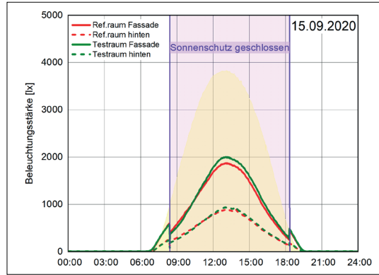
Abb. A90 Sonnenschutz und Beleuchtungsstärke (Cut-Off) am 15.09.2020 (IBP)
