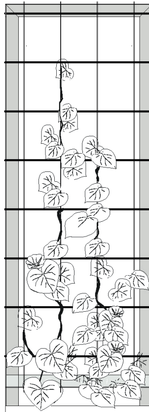
Abb. 52 Fassadenversuchsstand – Variante 4: Jakob Rope Systems, Ostfildern mit Pflanzplan (THN-AR) (Pflanzliste vgl. Tab. A13 im Appendix)
