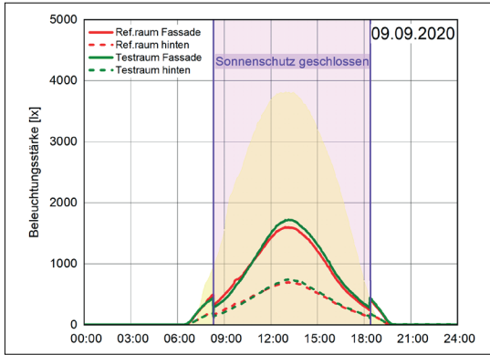
Abb. A89 Sonnenschutz und Beleuchtungsstärke (Cut-Off) am 09.09.2020 (IBP)
