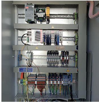
Abb. A6 Klemmkasten (THN-AR)
