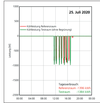
Abb. A54 Kühlleistung (Umluftkühlung) in den Zwillingräumen am 25. Juli 2020 (IBP)
