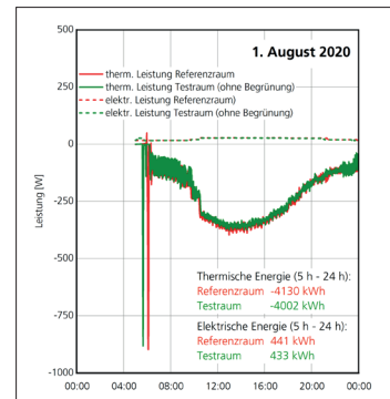
Abb. A60 Thermische (wasserseitig) und elektrische Leistung der DFL in den Zwillingräumen am 1. August 2020 (IBP)
