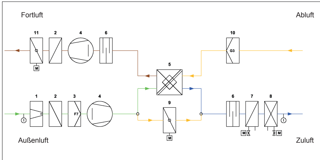
Abb. 55 Dezentrales Lüftungsgerät/ Funktionsschemata (THN-ieg) Aufbau und Funktion: Der Zuluftventilator (4) saugt im Primärluftbetrieb die Außenluft durch den Volumenstrombegrenzer (1), die Rückschlagklappe (2) und den Feinstaubfilter F7 (3) an, je nach Stellung der motorisierten Bypassklappe wird der Luftstrom (9) durch den rekuperativen Wärmerückgewinner (5) oder in energetisch sinnvollen oder durch den Geräteschutz bedingten Betriebsituationen durch den Bypass daran vorbei geleitet. Bei Bedarf wird die Luft im Wärmeüberträger gekühlt bzw. erhitzt. Danach strömt die Luft durch Schalldämpfer (6), Luftheizer (7) und Luftkühler (8) quellartig in den Innenraum.
