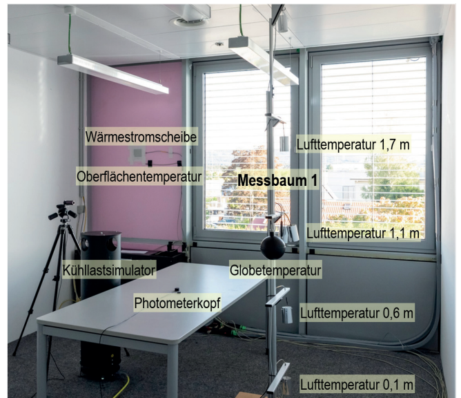
Abb. 87 Messaufbau in den Räumen. (IBP)
