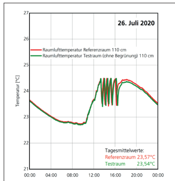
Abb. A56 Raumtemperatur (110 cm) in den Zwillingräumen am 26. Juli 2020 (IBP)
