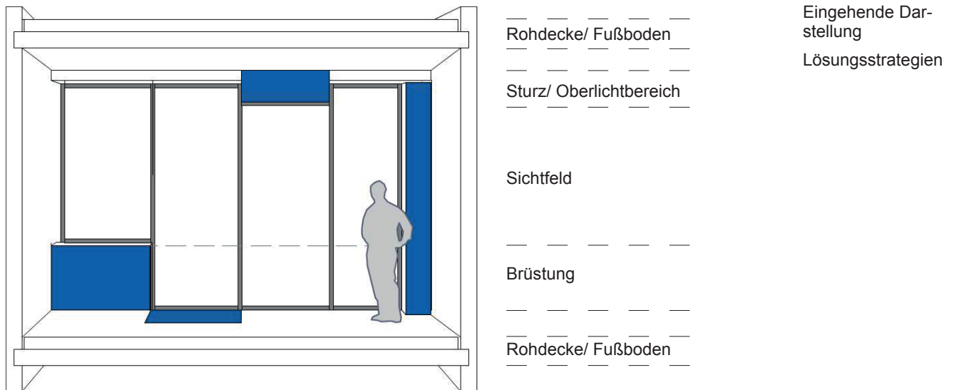
Abb. 7 Einbausituationen für DFL-Geräte mit Bezug zur vertikalen Zonierung von Fassaden (THN-AR)
