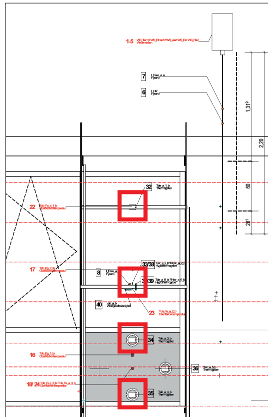
Abb. 13 Fassadenversuchsstand – Messpunkte für alternative Entnahmeorte (THN-AR)
