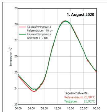
Abb. A59 Raumtemperatur (110 cm) in den Zwillingräumen am 1. August 2020 (IBP)
