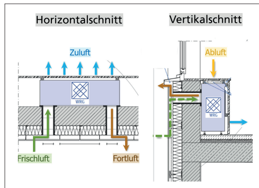
Abb. 75 Luften- und -auslässe des DFL-Gerätes (TROX 10/2016)
