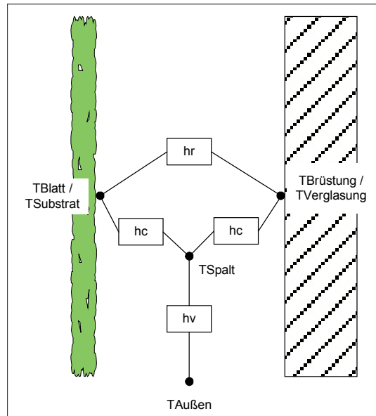
Abb. 17 Widerstandsnetzwerk für Mischsysteme und bodengebundene Systeme (THN-ieg)
