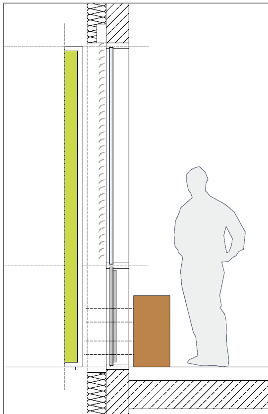
Abb. 12 Fassadenversuchsstand – Entnahmeorte der Zuluft (THN-AR)
