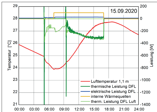
Abb. 101 Dezentrale Fassadenlüftungsgeräte – Referenzraum 15.09.2020 (IBP)
