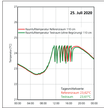
Abb. A53 Raumtemperatur (110 cm) in den Zwillingräumen am 25. Juli 2020 (IBP)
