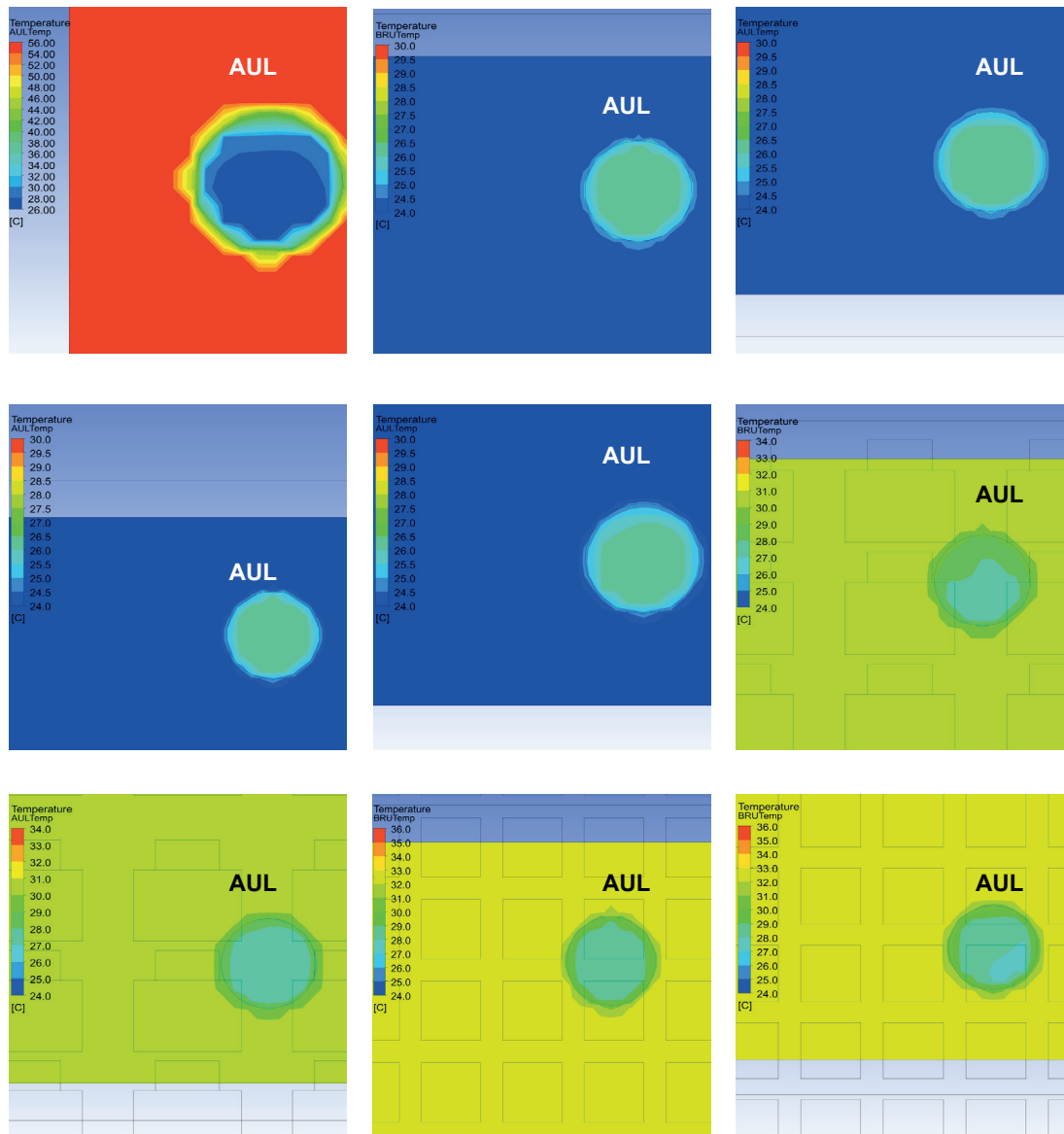
Abb. 23 – 31 Grenzschichttemperaturen für die untersuchten Systeme im Ansaugbereich (AUL) des Wetterschutzgitters der dezentralen Fassadenlüftung. Weiterhin sind die Brüstertemperaturen der Außenluftansaugung zu erkennen (alle THN-ieg) Ansaugtemperaturen
