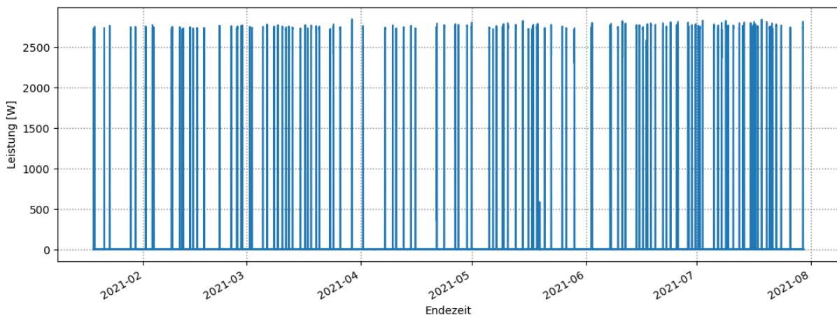
Abbildung 20: Ladelaastprofil E-Auto eines Haushalts
