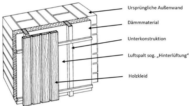
Abbildung 74: Wandaufbau mit hinterlüfteter Vorhangfassade [26]
