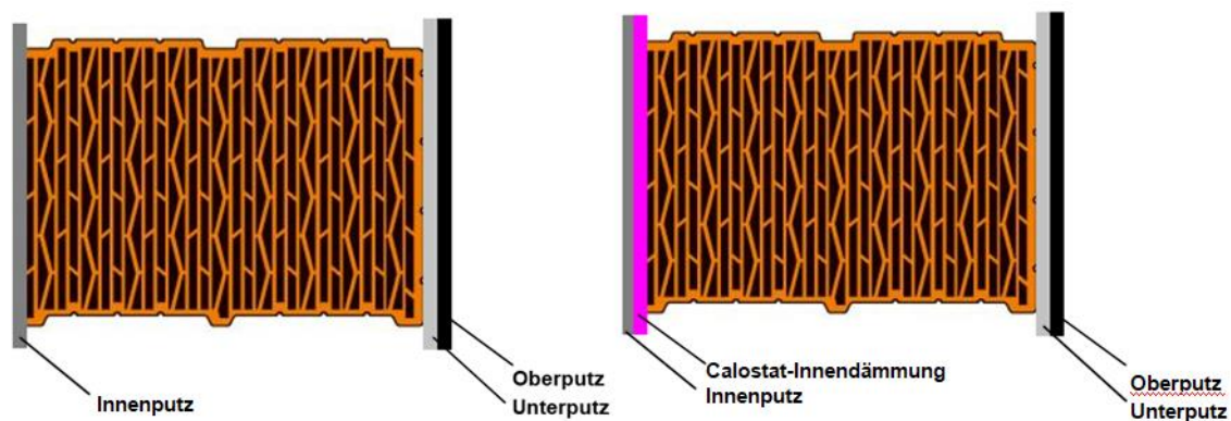
Abbildung 79: Schematischer Wandaufbau mit CALOSTAT® - Innendämmung, Innenputz sowie Ober- und Unterputz (rechts) im Vergleich mit einem gleichen Ziegel ohne CALOSTAT®, aber mit Innenputz, Unterputz und Oberputz (links)
